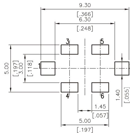
P.C.B. LAYOUT
